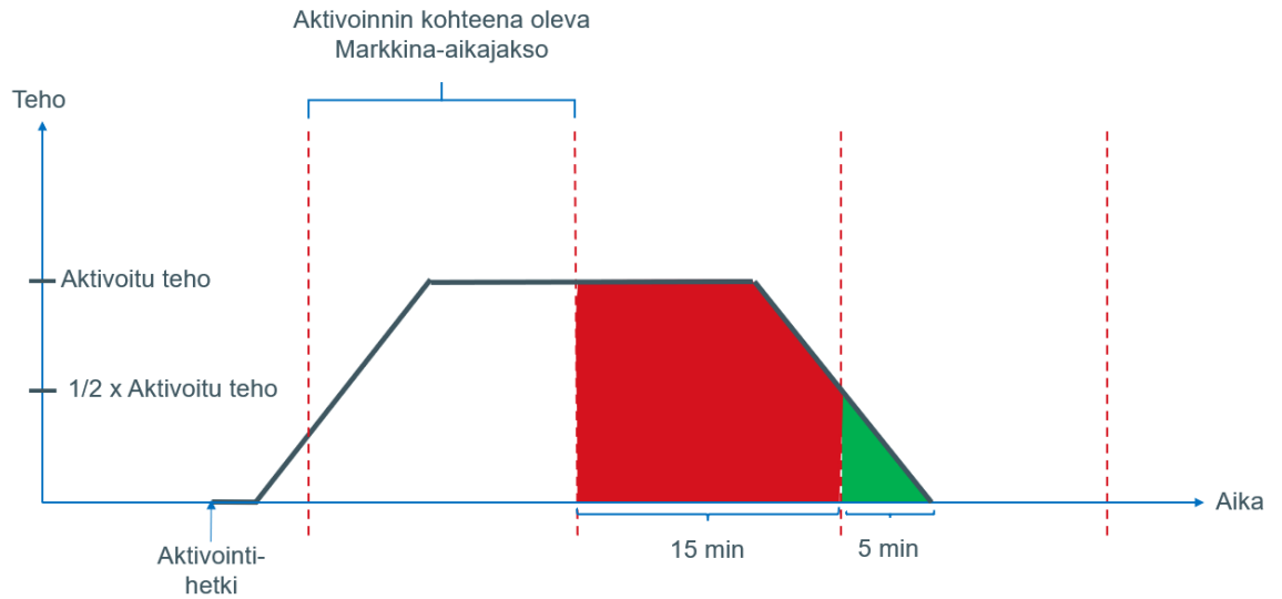
Kuva 9 Suoran aktivoinnin kohteena olevaa Markkina-aikajaksoa seuraavalle Taseselvitysjaksolle kohdistuva Aktivoidu säätöenergia, kun Tehomuutos alkaa ennen Suoran aktivoinnin kohteena olevaa Markkina-aikajaksoa, Suoran aktivoinnin kohteena olevan Markkina-aikajakson alussa tai sen aikana ja päättyy ennen sen loppua tai sen lopussa
