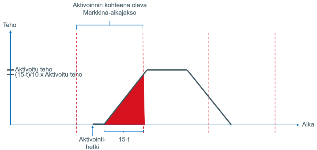
Kuva 8 Suoran aktivoinnin kohteena olevaa Markkina-aikajaksoa vastaavalle Taseselvitysjaksolle kohdistuva Aktivoitu säästöenergia, kun Tehonmuutos alkaa Suoran aktivoinnin kohteena olevan Markkina-aikajakson aikana ja päättyy seuraavalla Markkina-aikajaksolla
