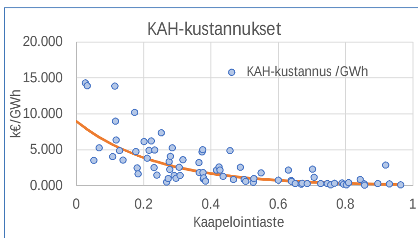
Kuva 4. KAH-kustannus kaapelointiasteen funktiona ja aineistoon sovittu malli.
