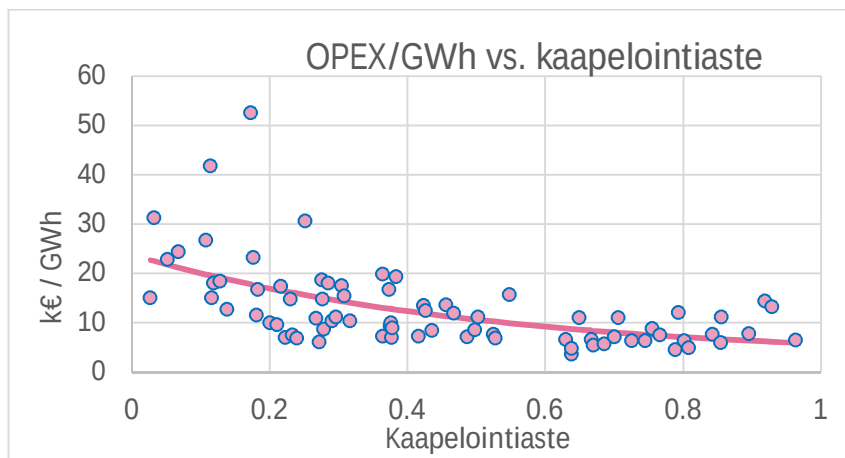
Kuva 32. Normeerattujen OPEX-kulujen ja kaapelipotentialin yhteys.
