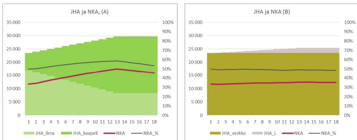
Kuva 13. Verkon jälleenhankinta-arvo (JHA) ja nykykäyttöarvo (NKA). A-tapauksessa (vas.) toimitusvarmuuden paranee kaapeliosuuden kasvulla, B-tapauksessa (oik.) nykyverkon varmuus parane paikallisin toimenpitein hankinta-arvoltaan JHA_L. JHA_verkko on nykyverkon jälleenhankinta-arvo.
