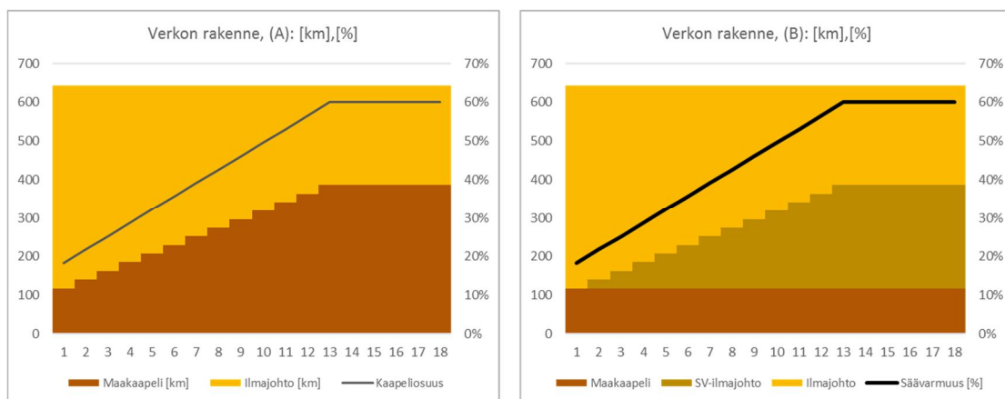
Kuva 12. Verkon rakenne, kun sovelletaan strategiaa A (vasen) ja strategiaa B (oikea). SV-ilmajohto tarkoittaa säävarmaa ilmajohtoa, joka on toteutettu lokaalein toimenpitein. Toimintaohjelma muodostuu kaapeliosuuden/säävarman verkon osuuden kasvattamisesta 18 %:sta 60 %:iin 12 vuodessa.
