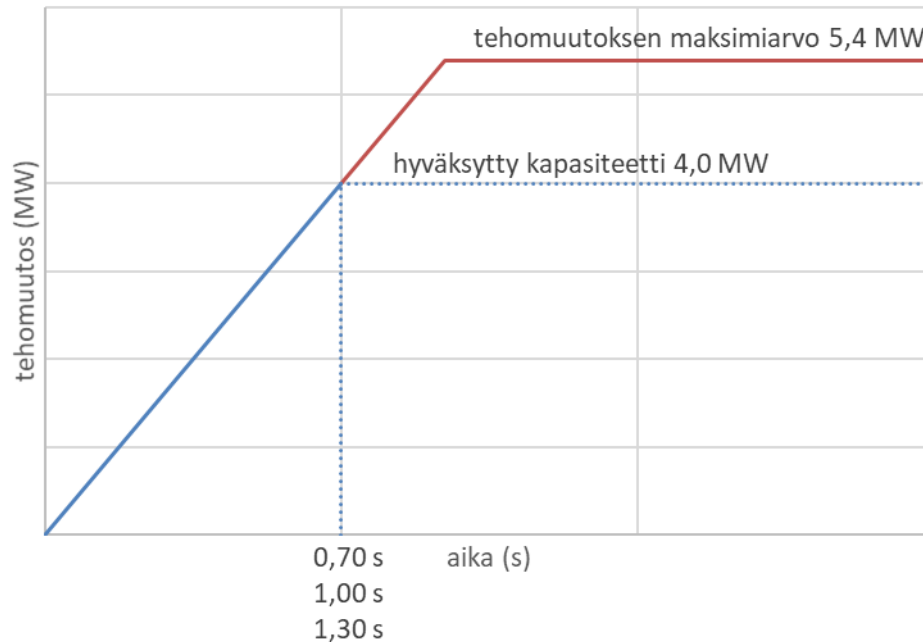
Kuva 3.1 Suurin sallittu aktivoituvaa tehoa suhteessa hyväksyttyyn kapasiteettiin
