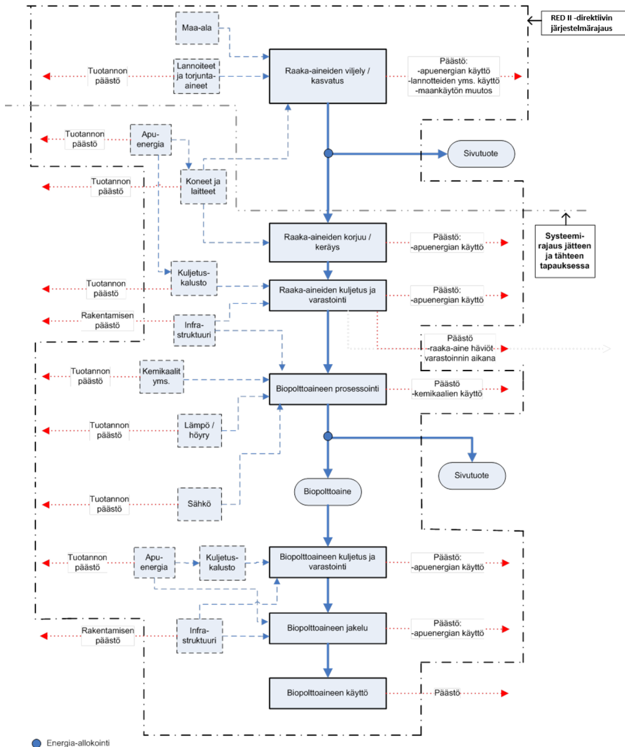
KUVA 3 RED II-DIREKTIIVIN JÄRJESTELMÄRAJAU
