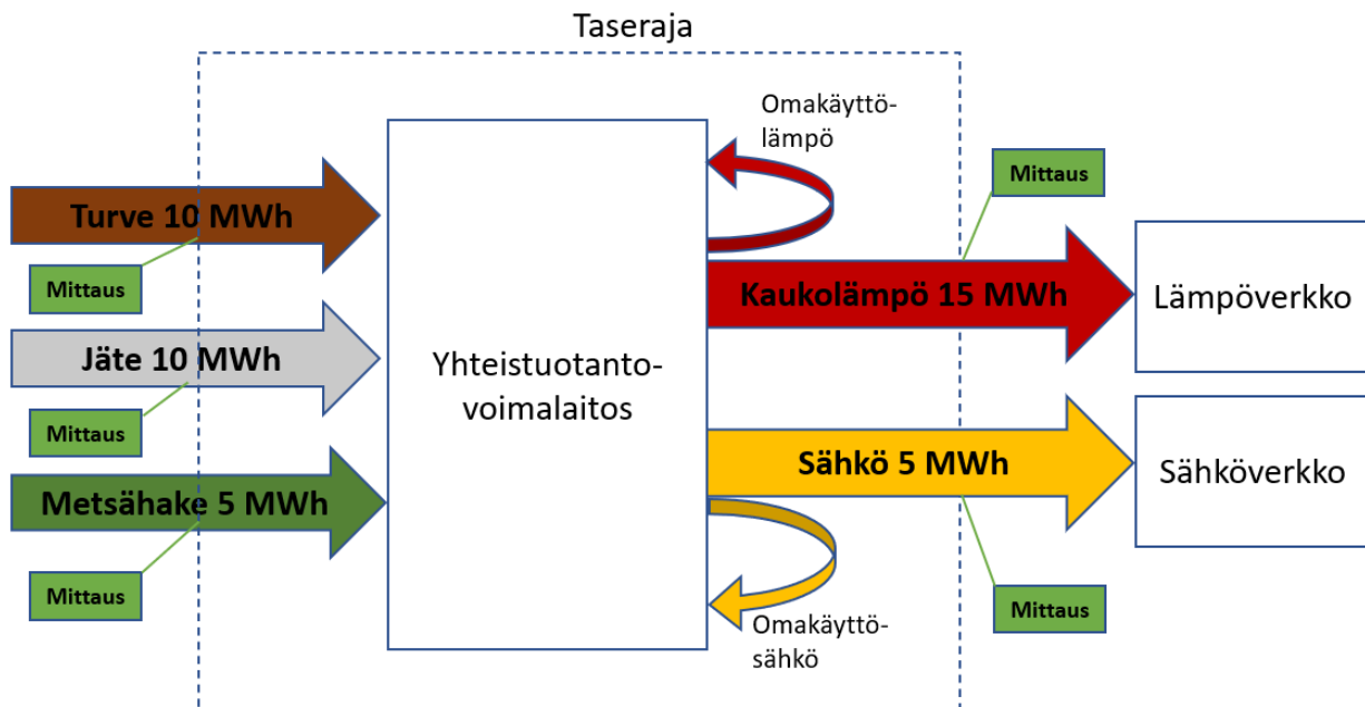
Kuva 6. Esimerkki monipolttoainelaitoksesta.
